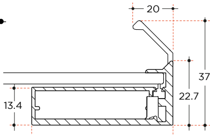
Sezione maniglia / Handle section
