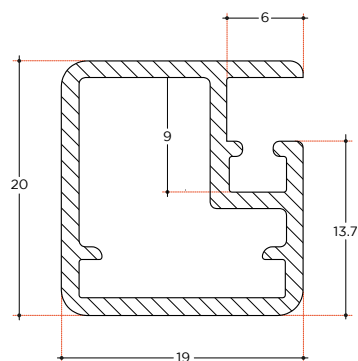
Sezione / Section
