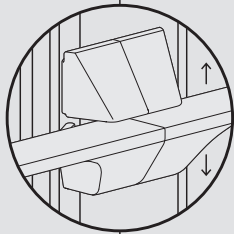
Aggancio per accessori riposizionabili sulla lunghezza del profilo / Accessories that can be repositioned along the length of the profile
