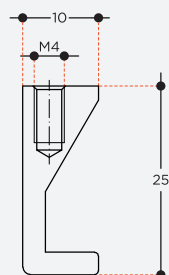
SEZIONE A-A /SECTION
