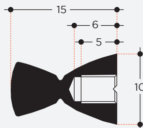
SEZIONE A-A /SECTION
