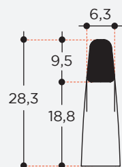
SEZIONE A-A /SECTION
