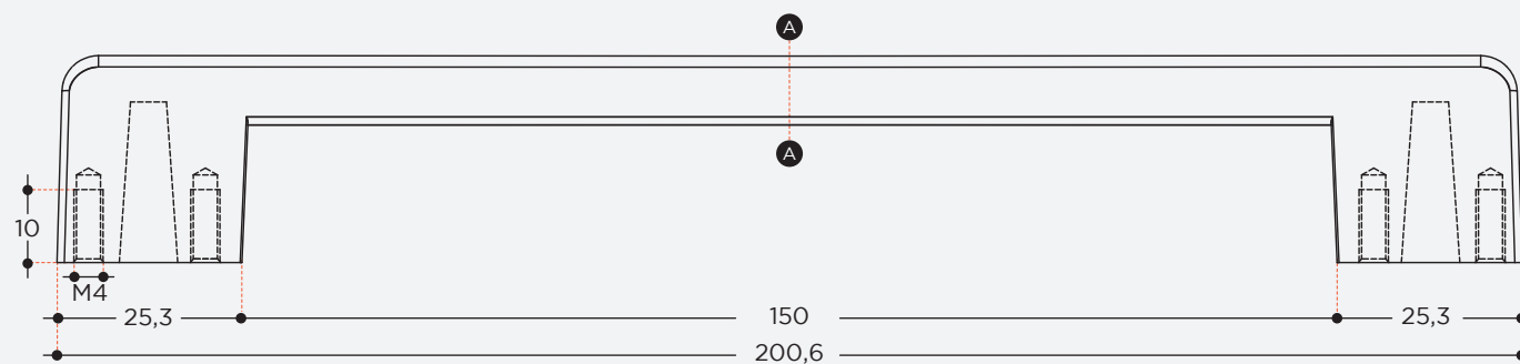
SEZIONE A-A /SECTION
